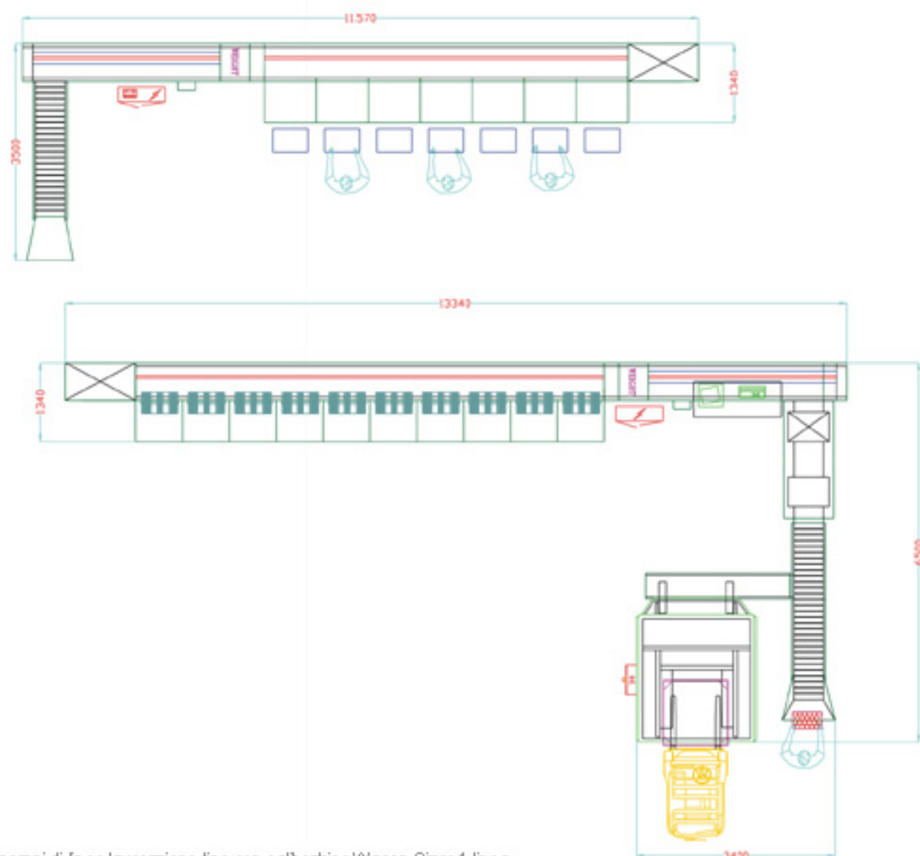
Esempi di linee lavorazione tipo con calibratrice Wagon Sizer 1 linea
