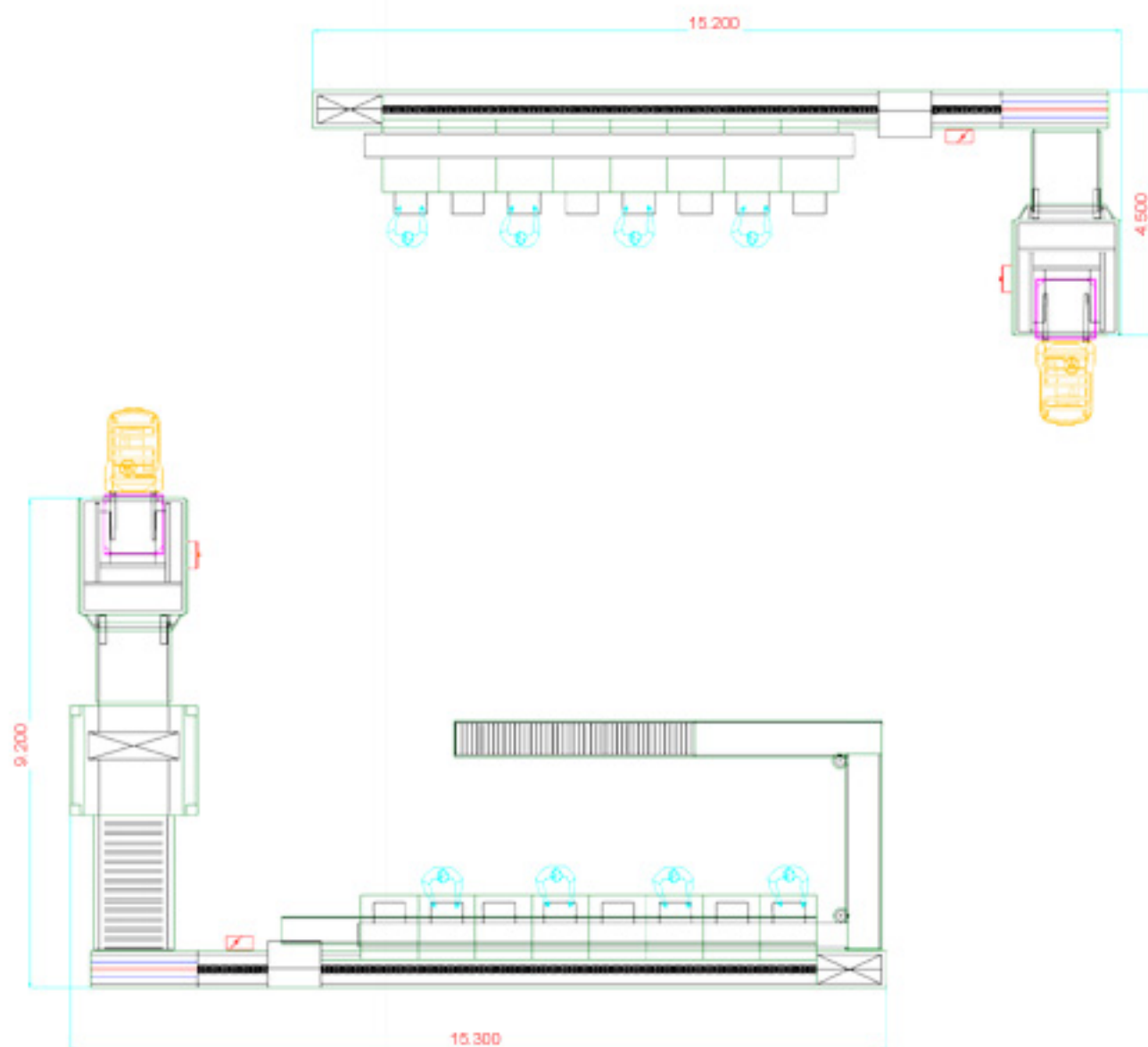
Esempi di linee lavorazione tipo con calibratrice Big Cup Sizer
